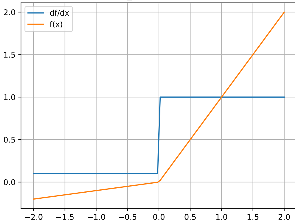
leaky_relu(x, slope=0.1)
